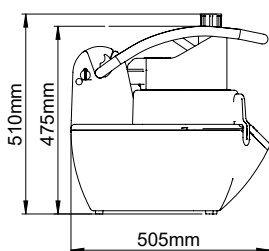
POHĽAD ZBOKU
