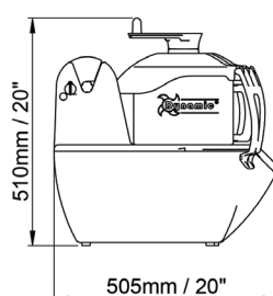
POHĽAD ZBOKU
