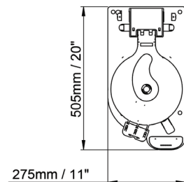
POHĽAD ZVRCHU
