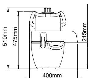
POHĽAD SPREDU
